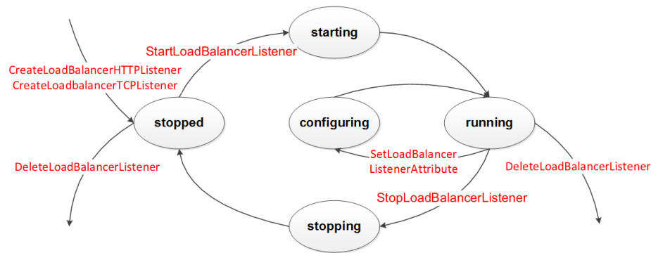
负载均衡 Listener状态转换图
