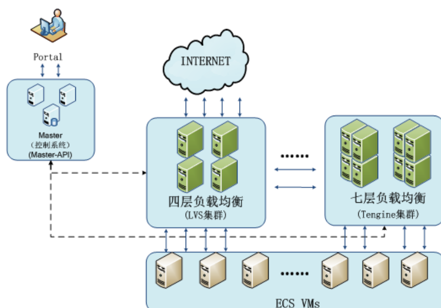
SLB集群模块、组件图
